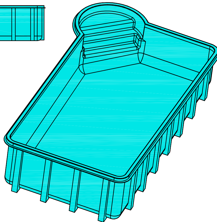
PISCINA MODELO CARIBE DIMENSIONES: 6,25 x 3,20 x 1,10-1,50 m
