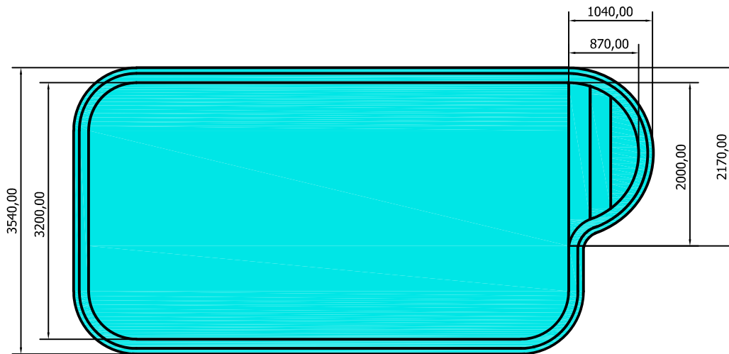
PISCINA MODELO CAPRICHIO DIMENSIONES: 6,90 x 3,20 x 1,10-1,50 m
