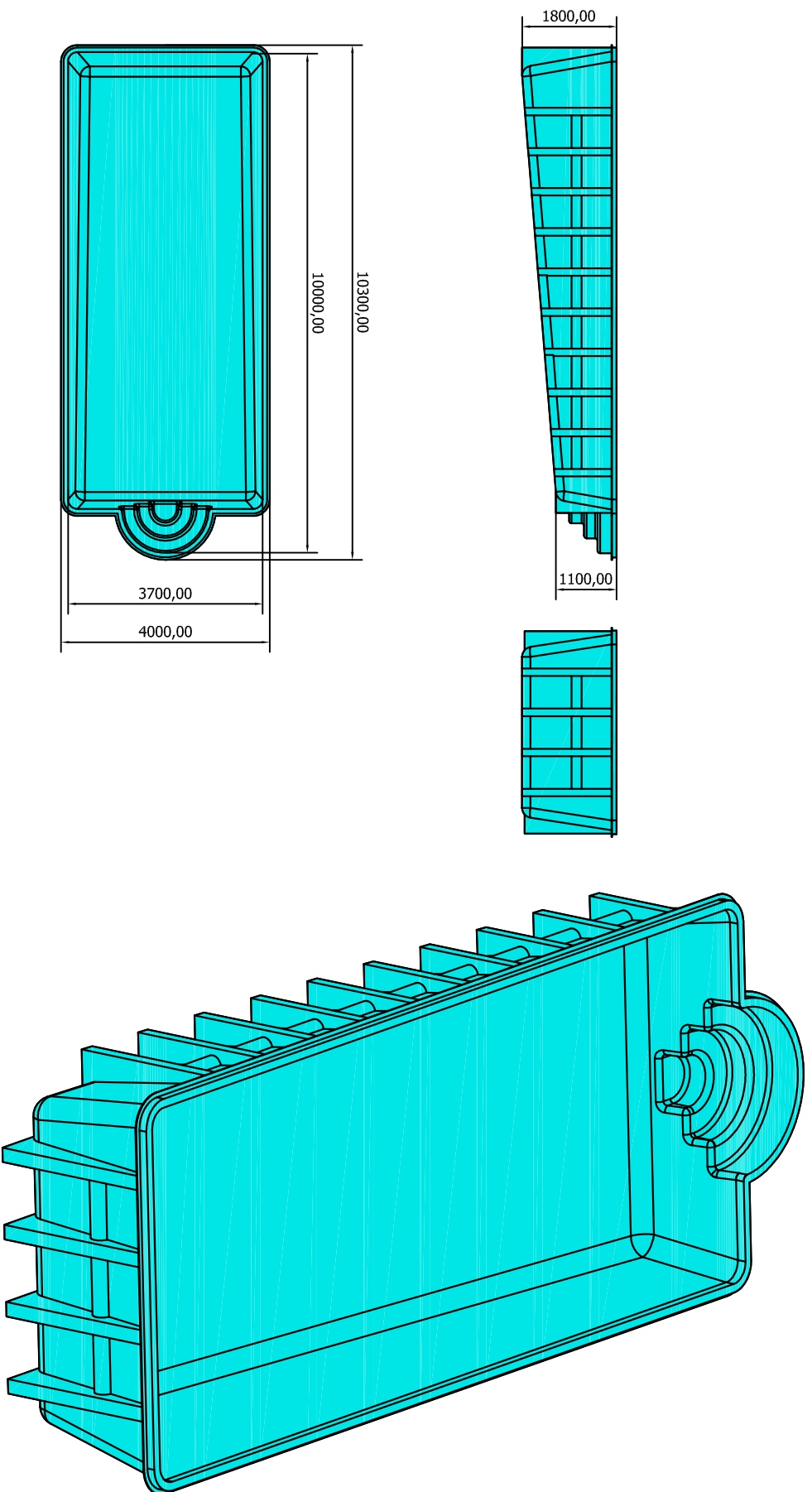
PISCINA MODELO ZAFIRO DIMENSIONES: 10,00 x 3,70 x 1,10-1,80 m
